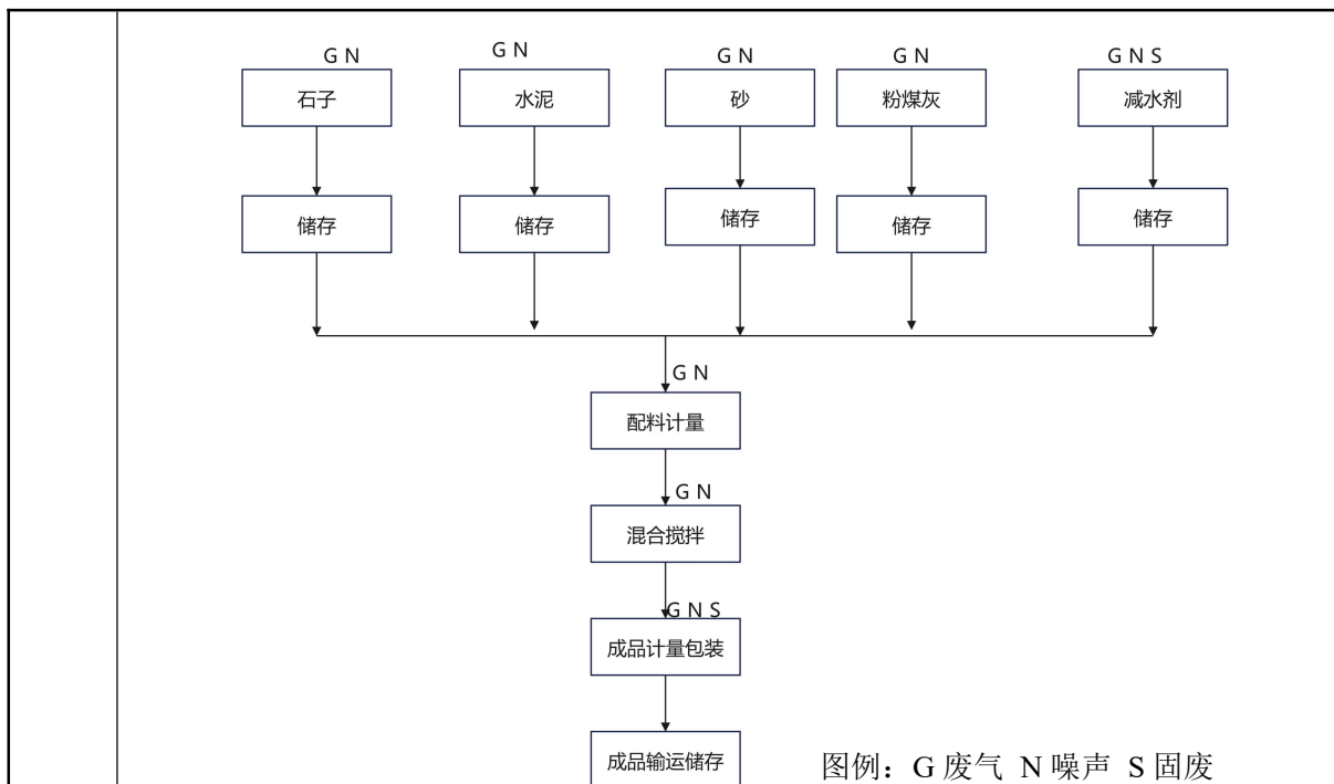
图2 营运期工艺流程及排污节点图
